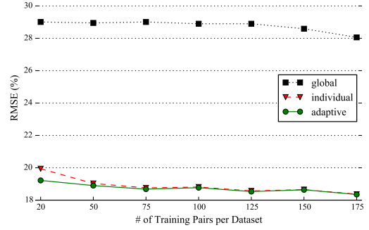
(b) Error.
